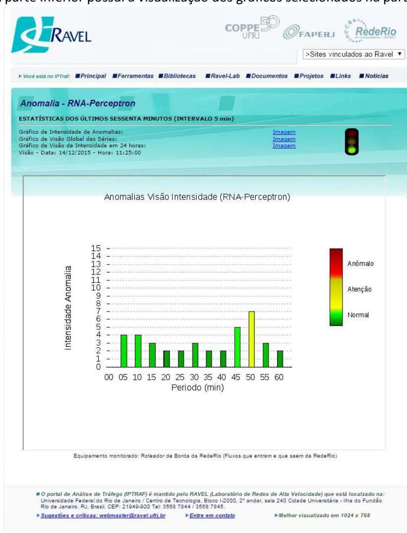
Figura 2: Interface gráfica Web do Módulo Anomalia baseado em Inteligência Artificial
