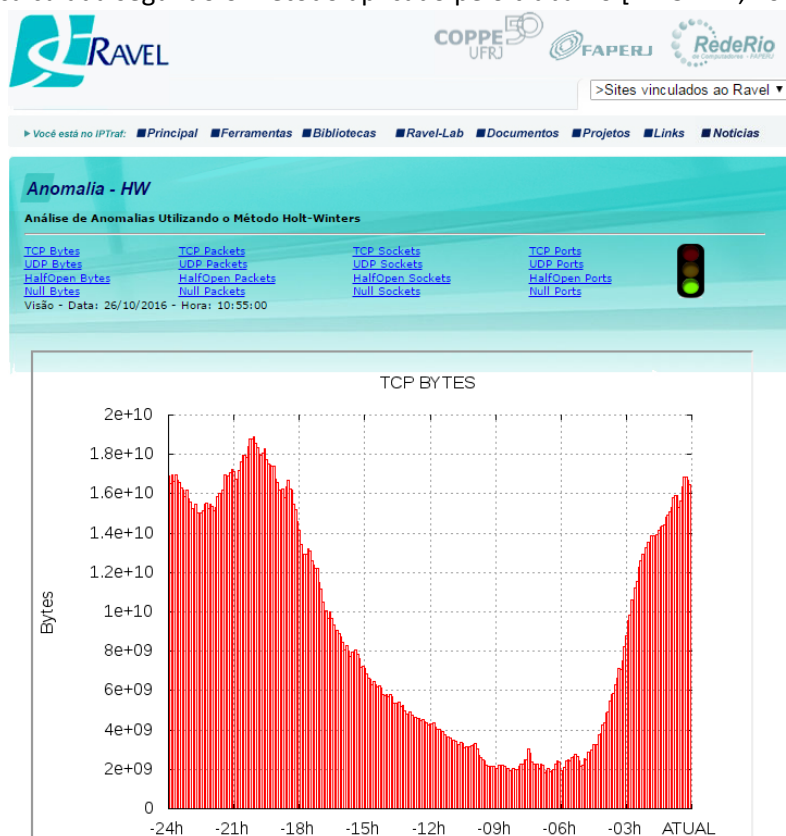
Figura 1: Interface gráfica Web do Módulo Anomalia baseado em Séries Temporais
